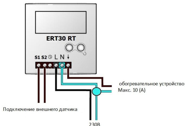
Схема подключения 2
