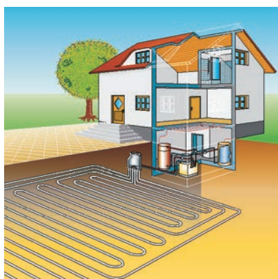
Схема прибора - Земляной коллектор
